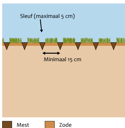
Zodebemester, mest komt een paar centimeter diep in de bodem Foto: Veenhuis bv.
