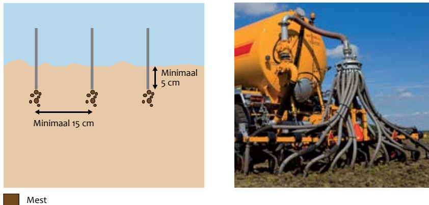
Bouwlandinjecteur Foto: Veenhuis bv.
