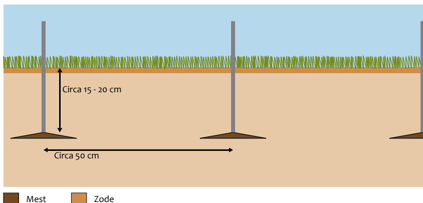
Mestinjectie, mest komt in brede sleuven op 15-20 cm diepte.
