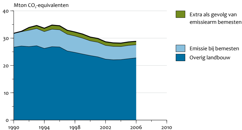
Broeikasgasemissies uit de landbouw met het emissieverhogende effect (koolstofdioxide en lachgas) van emissie-arm bemesten hierop.
