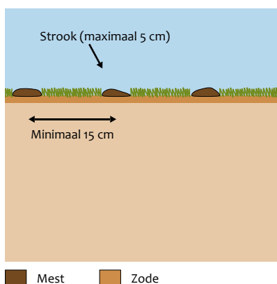
Sleepvoetbemester, mest wordt tussen het gras gedeponeerd Foto: Schuitemaker Machines bv.
