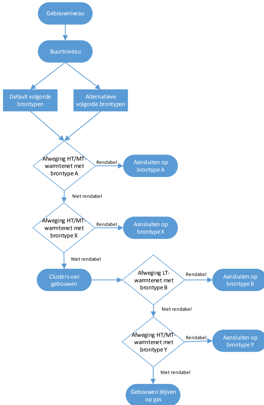
Figuur 19 - Stroomdiagram werkwijze berekenen gebiedsmaatregelen in Vesta MAIS
