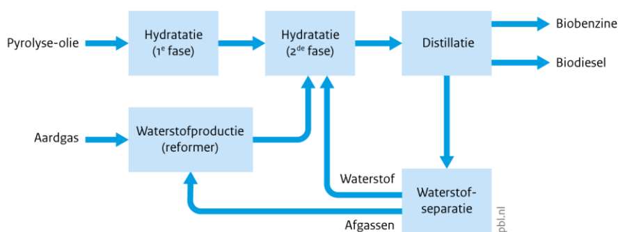
Figuur 10.3 Opwaarderding pyrolyse-olie met geïntegreerde waterstofproductie
