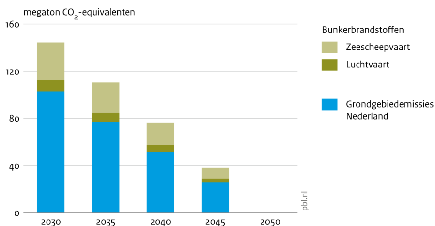
Figuur 2.2 Broeikasgasemissiedoelen
